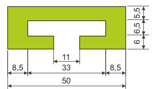
C 41 PERFIL DISCONTINUADO // REEMPLAZADO POR PERFIL C43
