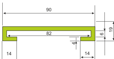
C Clip
