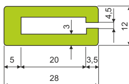
U Clip 35
