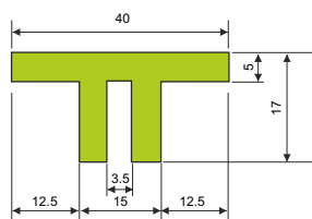
Uπ 35
