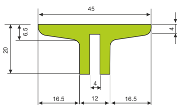
Uπ 45
