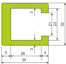
U Clip 26
