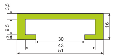
C 52/80
