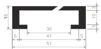
C 41 PERFIL DISCONTINUADO // REEMPLAZADO POR PERFIL C43
