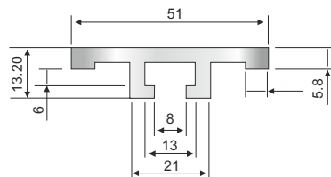
PERFIL AL. 50x6
