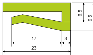
L Clip
