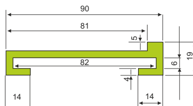
C 82 L
