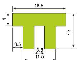
Uπ 40 con GUIA
