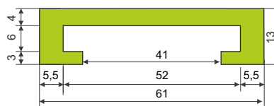
C 52
