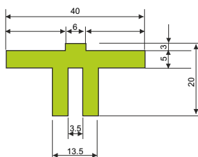
Uπ 45
