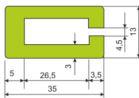
U Clip 35
