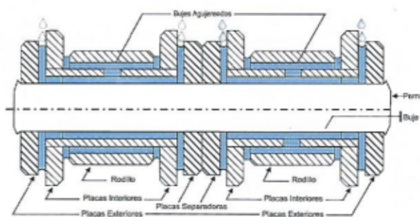
Corte transversal de una cadena "Star Chain" múltiple, mostrando bujes agujereados en el centro y juntas exageradas.
