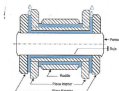
Corte transversal de una cadena standard mostrando juntas exageradas.
