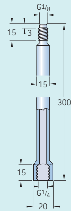
Tubo alargador de rosca G 1 / 8
