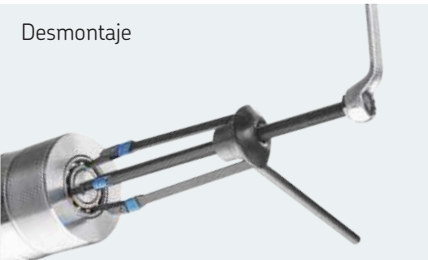
Desmontaje
