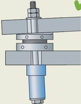
Tornillo recto
