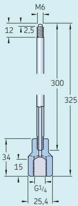
Tubo alargador de rosca M6 con racor de conexión
