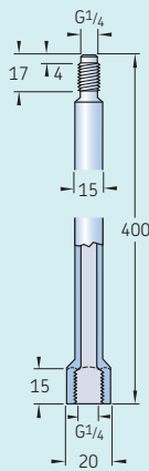
Tubo alargador de rosca G 1 / 4
