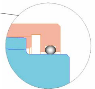
CIERRE POR O'RING
